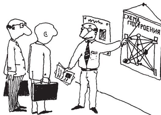
Построение функций принадлежности...
