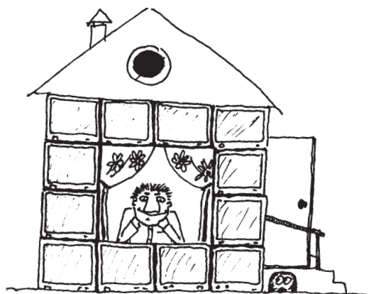
Методы наименьших квадратов...
